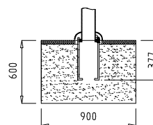
E: 1/50
